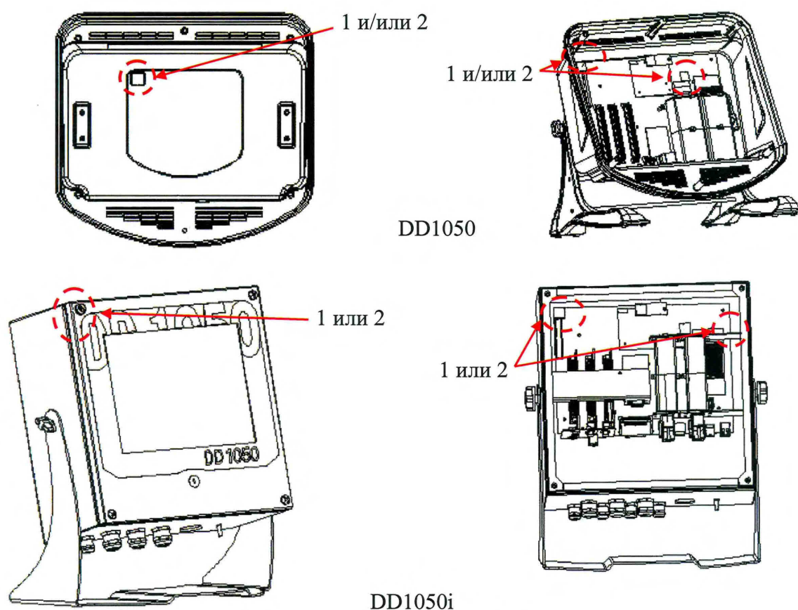
Рисунок 6 - Схемы пломбировки
